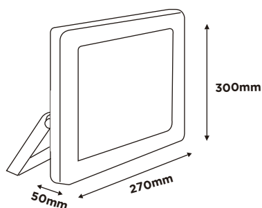
REFLECTOR
